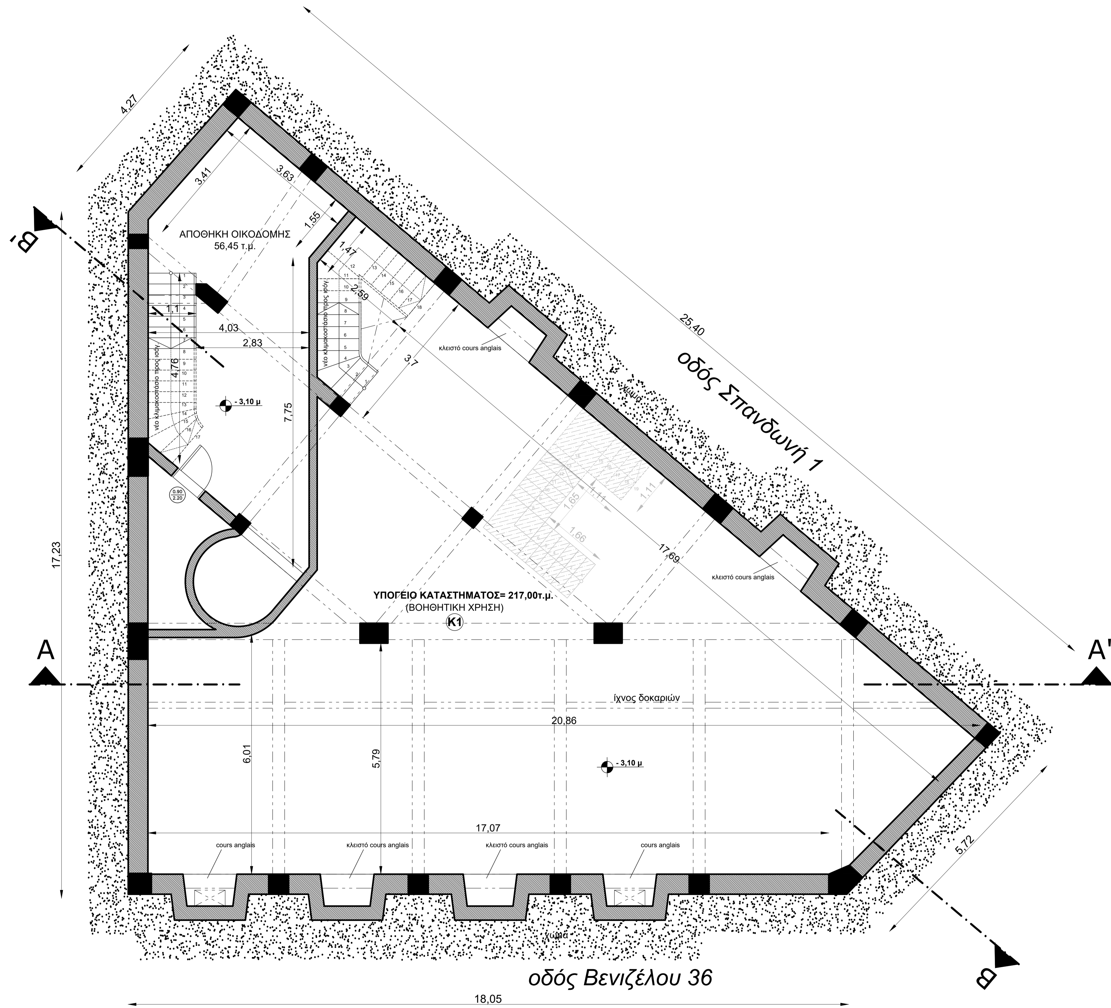
ΚΑΤΟΨΗ ΥΠΟΓΕΙΟΥ
